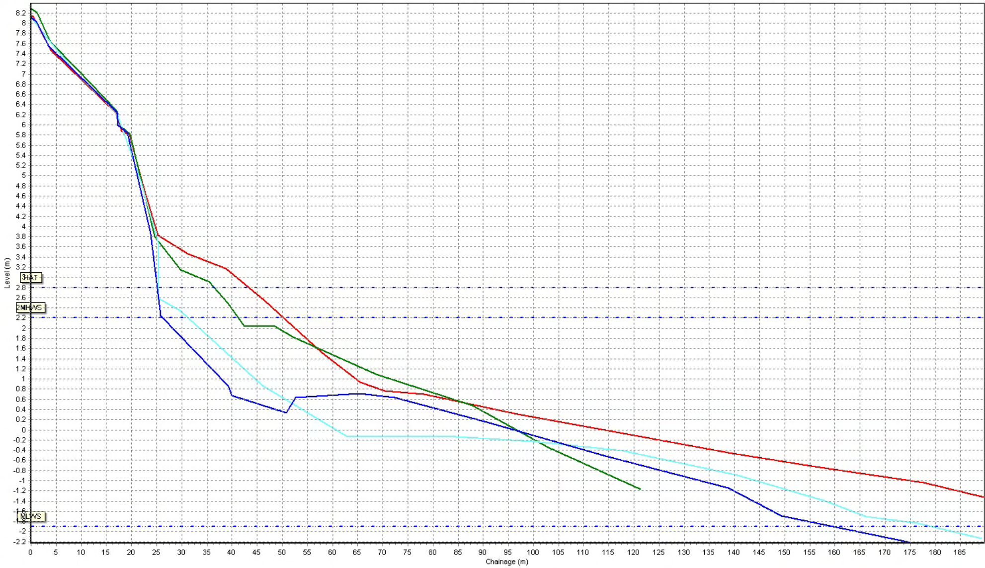
Beach Profiles: 1aBTBC09
