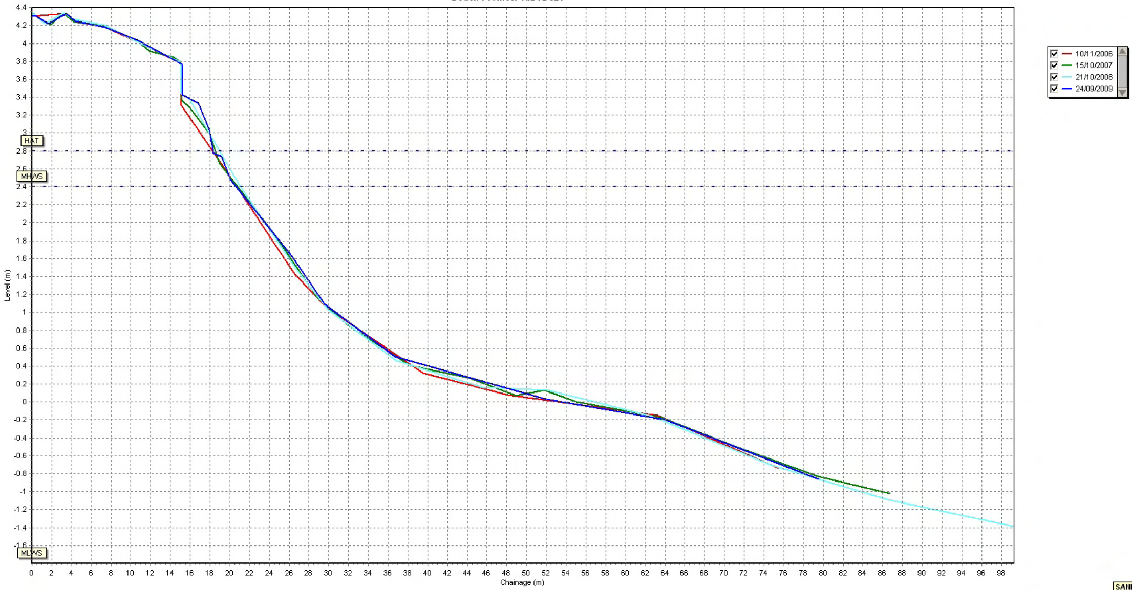
Beach Profiles: 1aBTBC24
