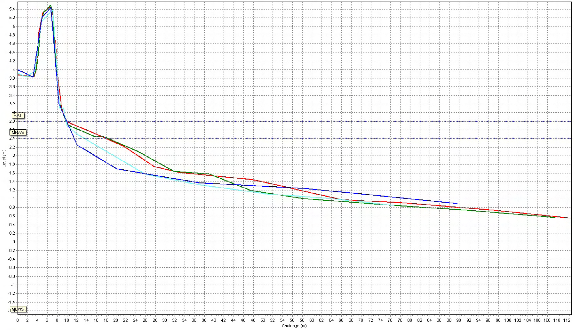
Beach Profiles: 1aBTBC32
