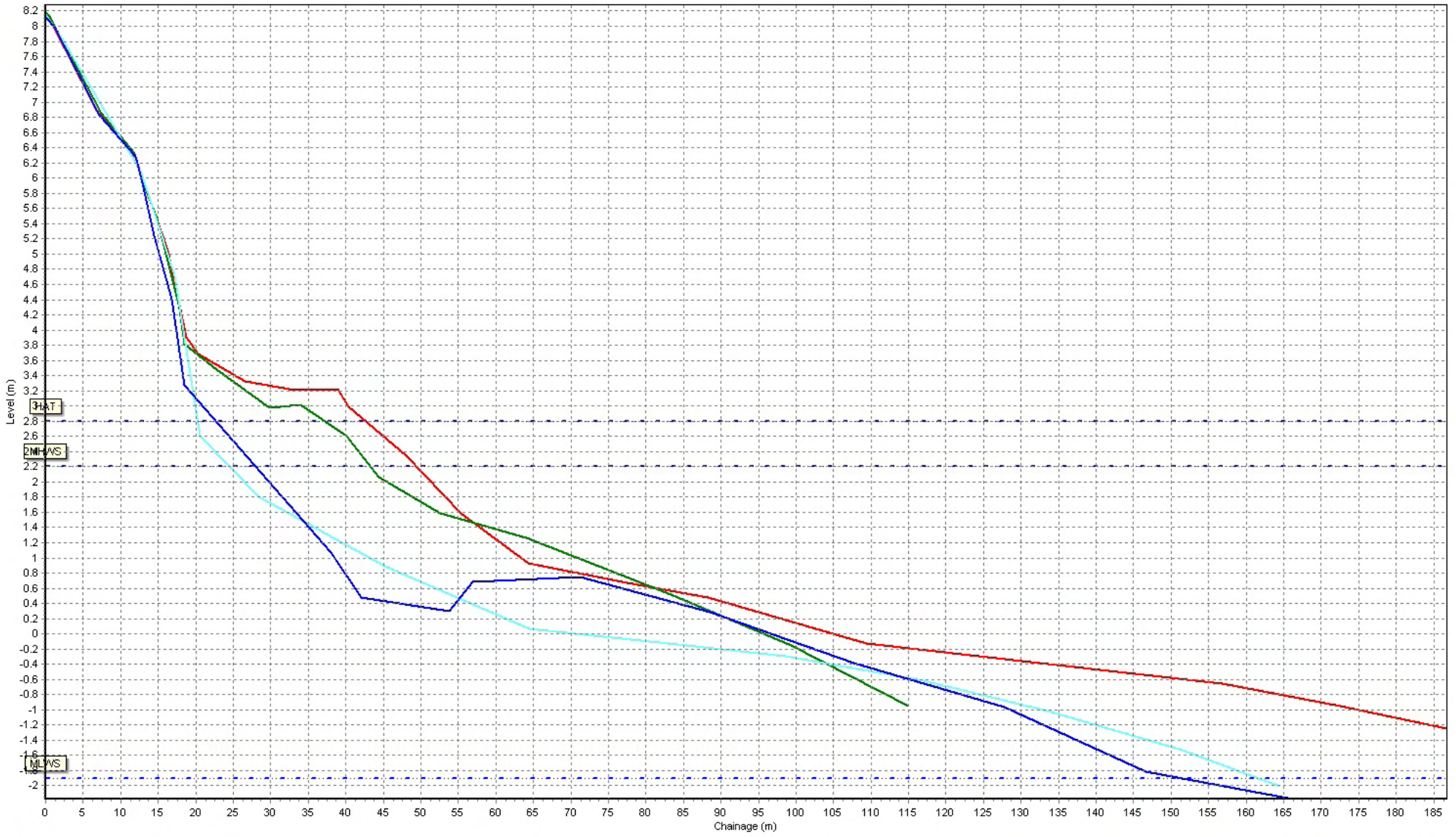
Beach Profiles: 1aBTBC10
