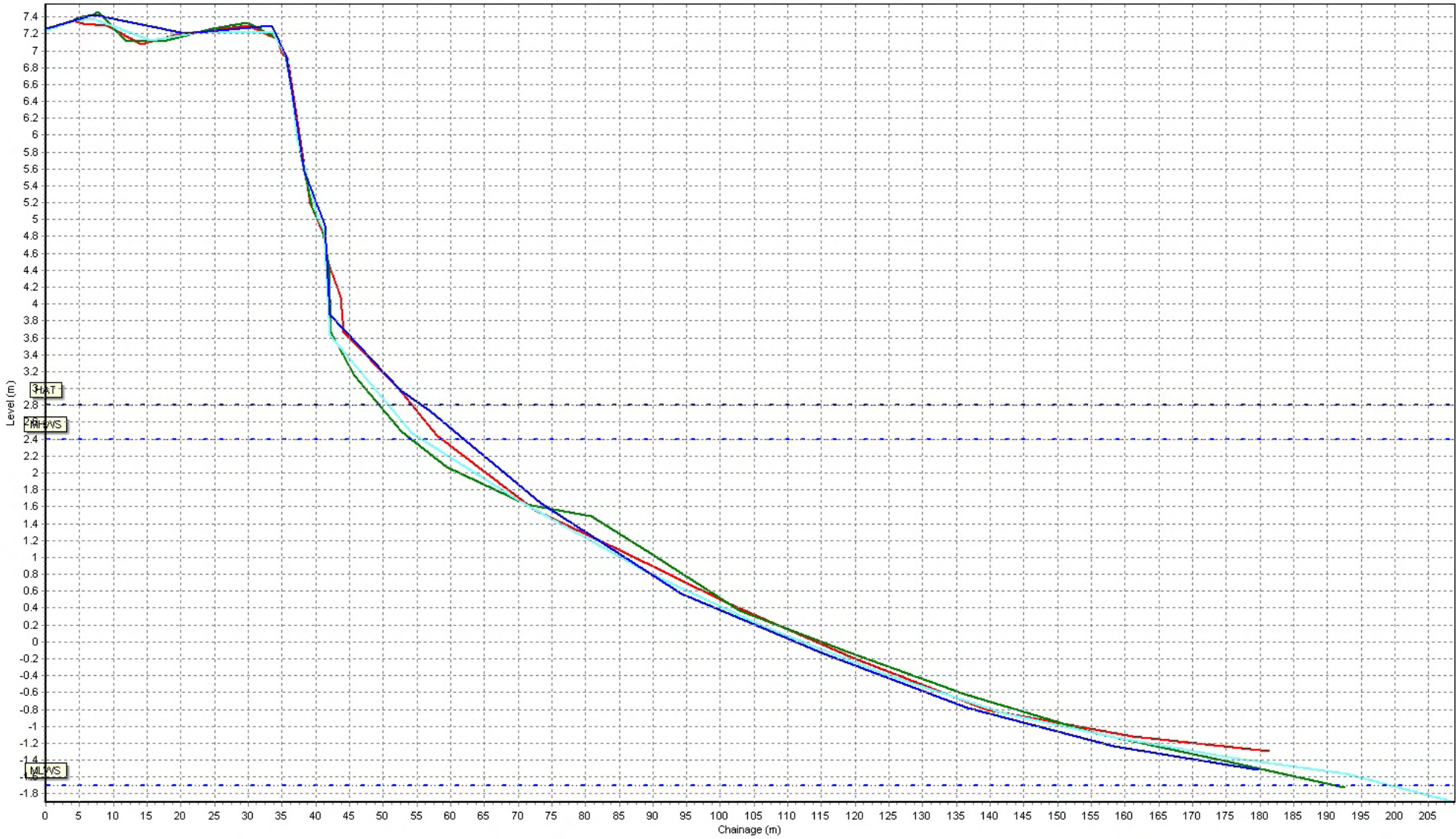
Beach Profiles: 1aBTBC30
