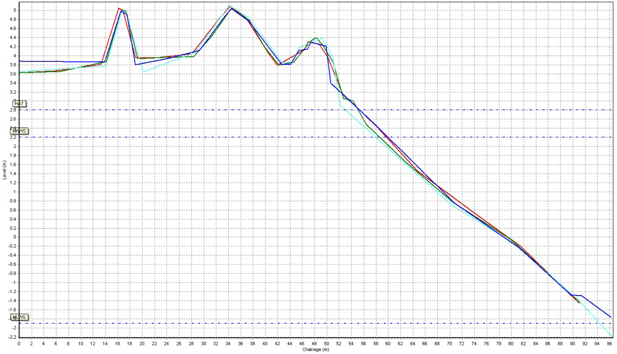
Beach Profiles: 1aBTBC03
