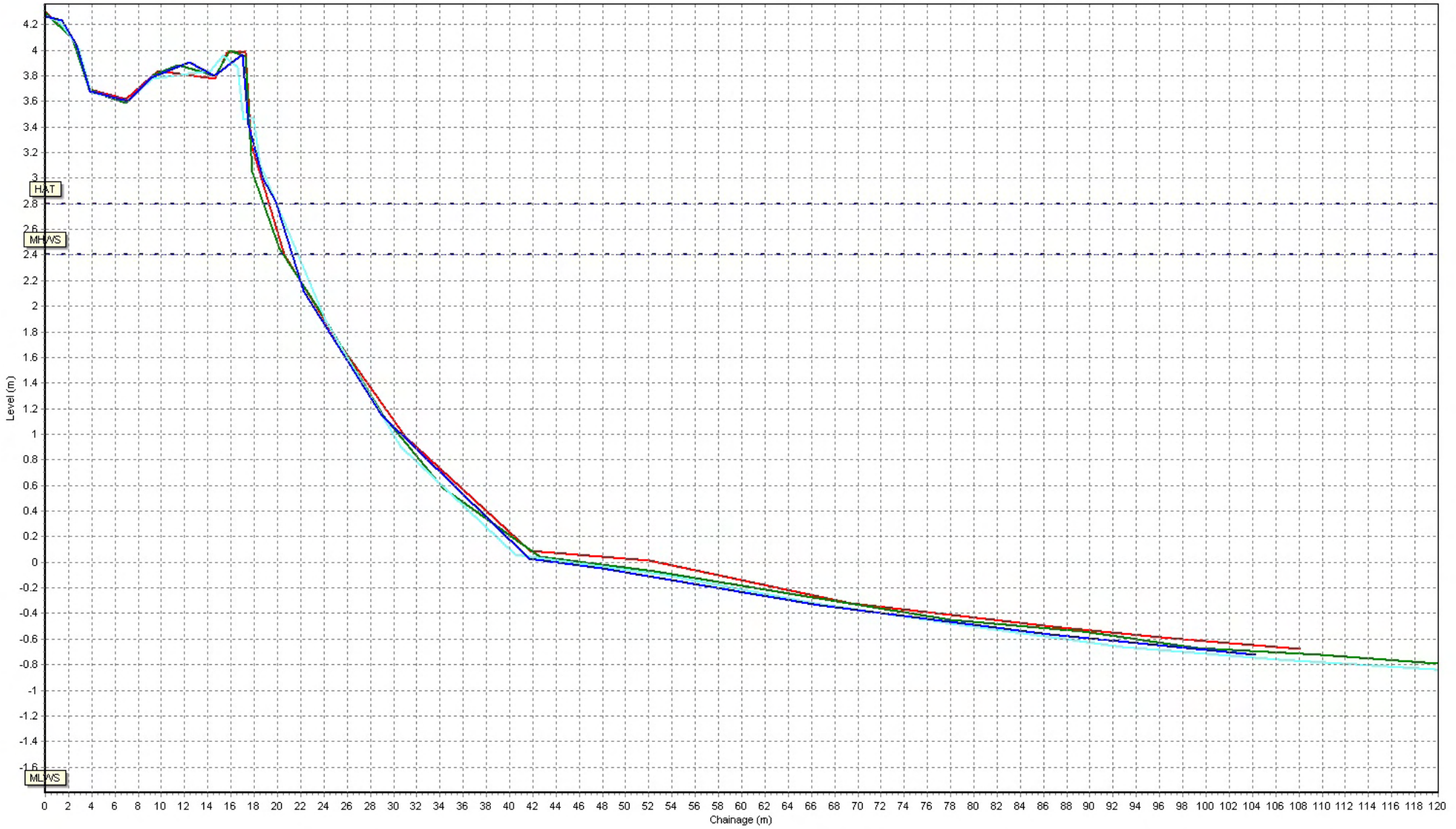
Beach Profiles: 1aBTBC25
